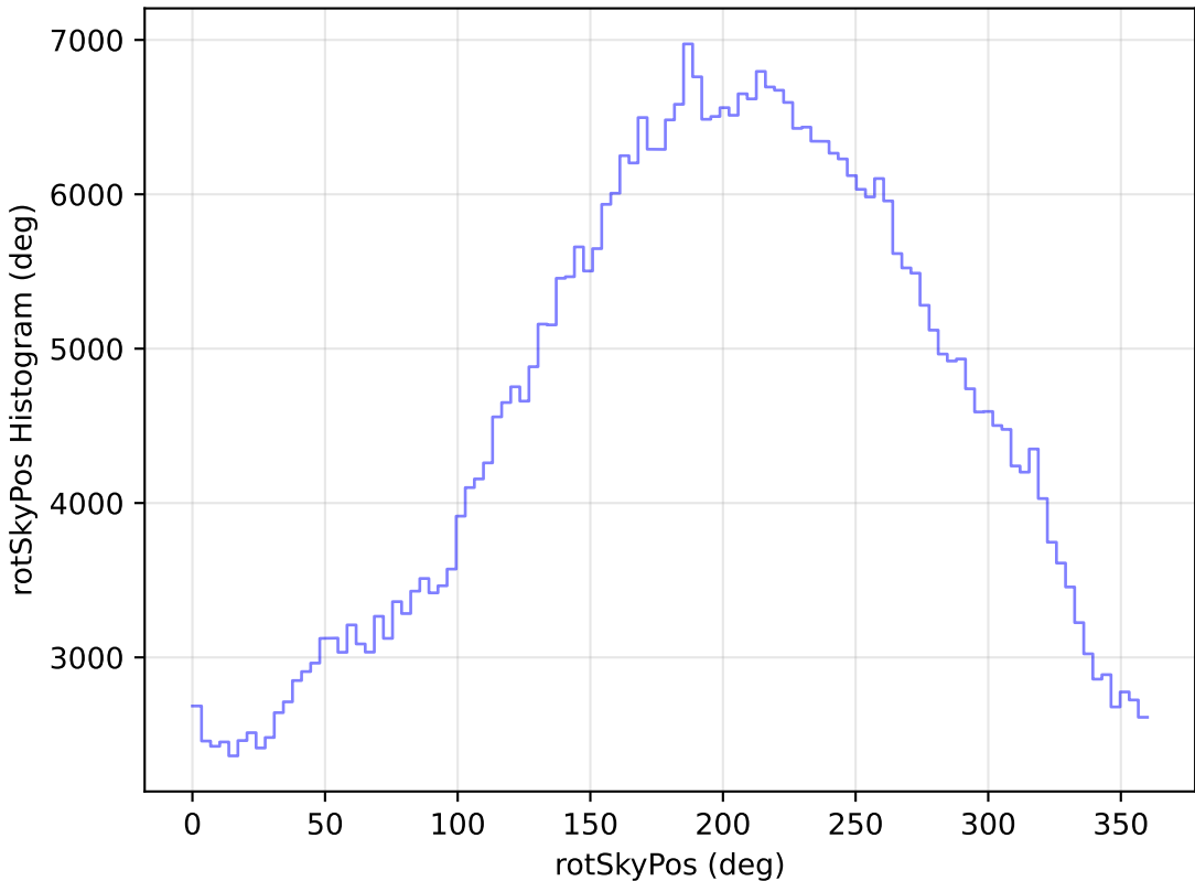
too_elab_r256_d3_ugrizy_v3.4_10yrs All sky r band: rotSkyPos Histogram
