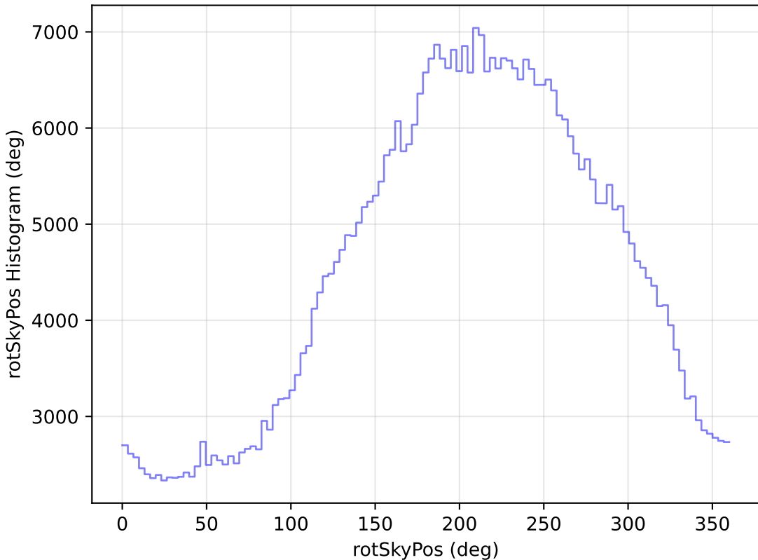
too_elab_r256_d3_ugrizy_v3.4_10yrs All sky i band: rotSkyPos Histogram
