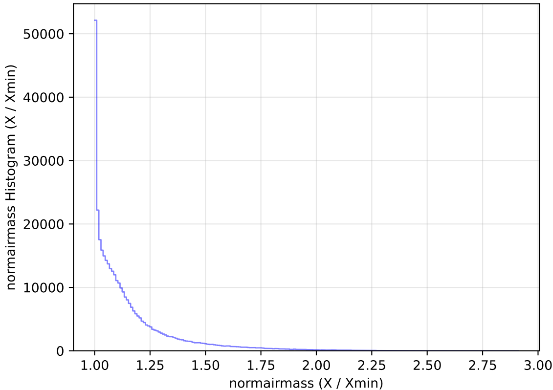
too_elab_r256_d3_ugrizy_v3.4_10yrs WFD y band: normairmass Histogram
