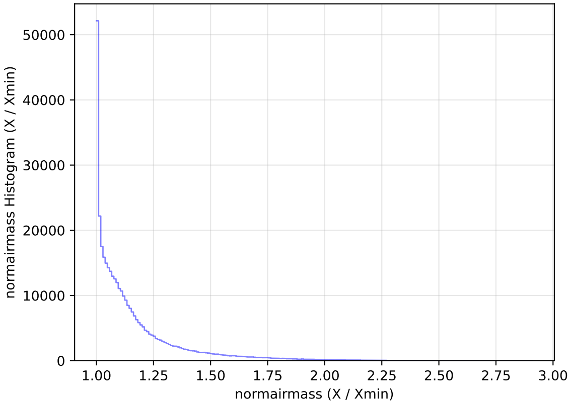
too_elab_r256_d3_ugrizy_v3.4_10yrs All sky y band: normairmass Histogram
