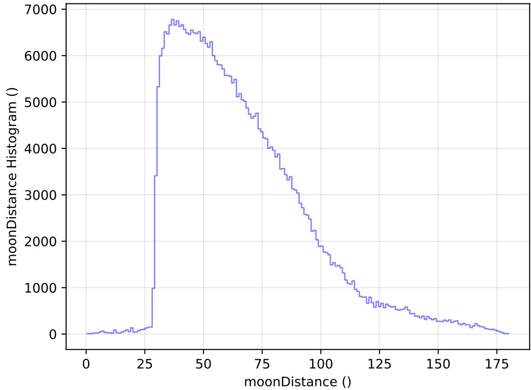
too_elab_r256_d3_ugrizy_v3.4_10yrs WFD y band: moonDistance Histogram
