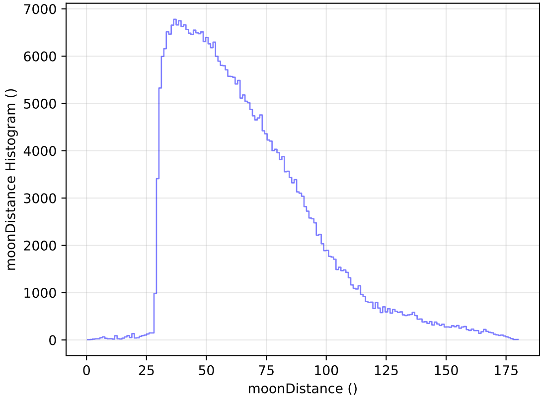
too_elab_r256_d3_ugrizy_v3.4_10yrs All sky y band: moonDistance Histogram
