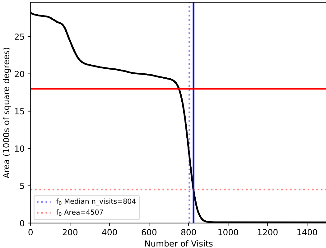
too_elab_r256_d3_ugrizy_v3.4_10yrs All sky: f0
