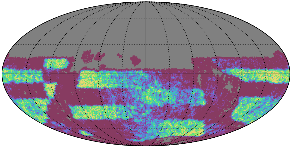
too_elab_r256_d3_ugrizy_v3.4_10yrs Yr 3-4 y band: NVisits
