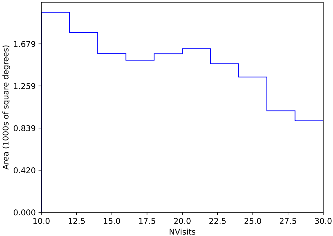
too_elab_r256_d3_ugrizy_v3.4_10yrs Yr 3-4 y band: NVisits
