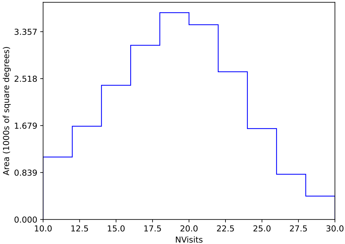
too_elab_r256_d3_ugrizy_v3.4_10yrs Yr 1 y band: NVisits
