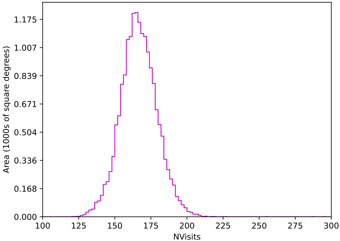
too_elab_r256_d3_ugrizy_v3.4_10yrs WFD z band: NVisits
