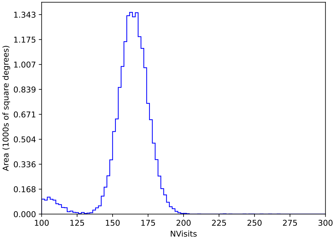
too_elab_r256_d3_ugrizy_v3.4_10yrs WFD y band: NVisits
