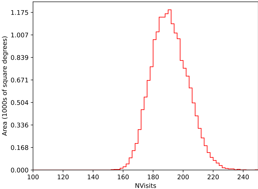
too_elab_r256_d3_ugrizy_v3.4_10yrs WFD i band: NVisits
