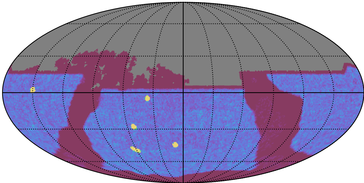
too_elab_r256_d3_ugrizy_v3.4_10yrs All sky y band: NVisits
