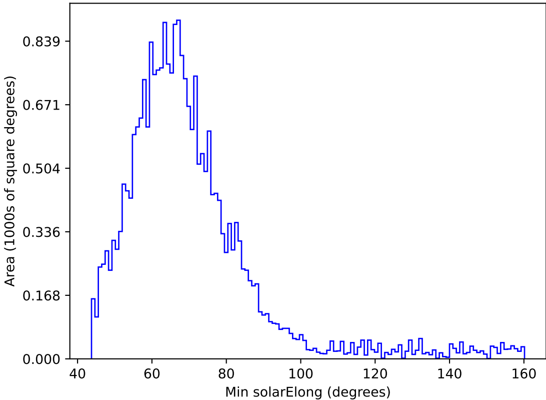
too_elab_r256_d3_ugrizy_v3.4_10yrs All sky y band: Min solarElong
