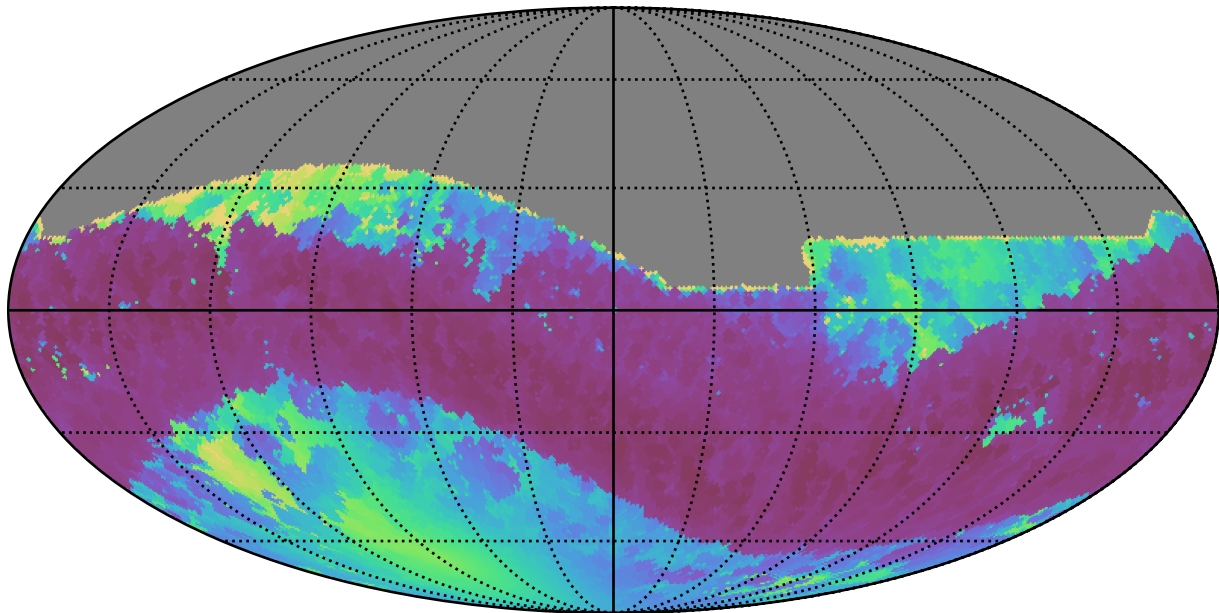
too_elab_r256_d3_ugrizy_v3.4_10yrs All sky i band: Min solarElong
