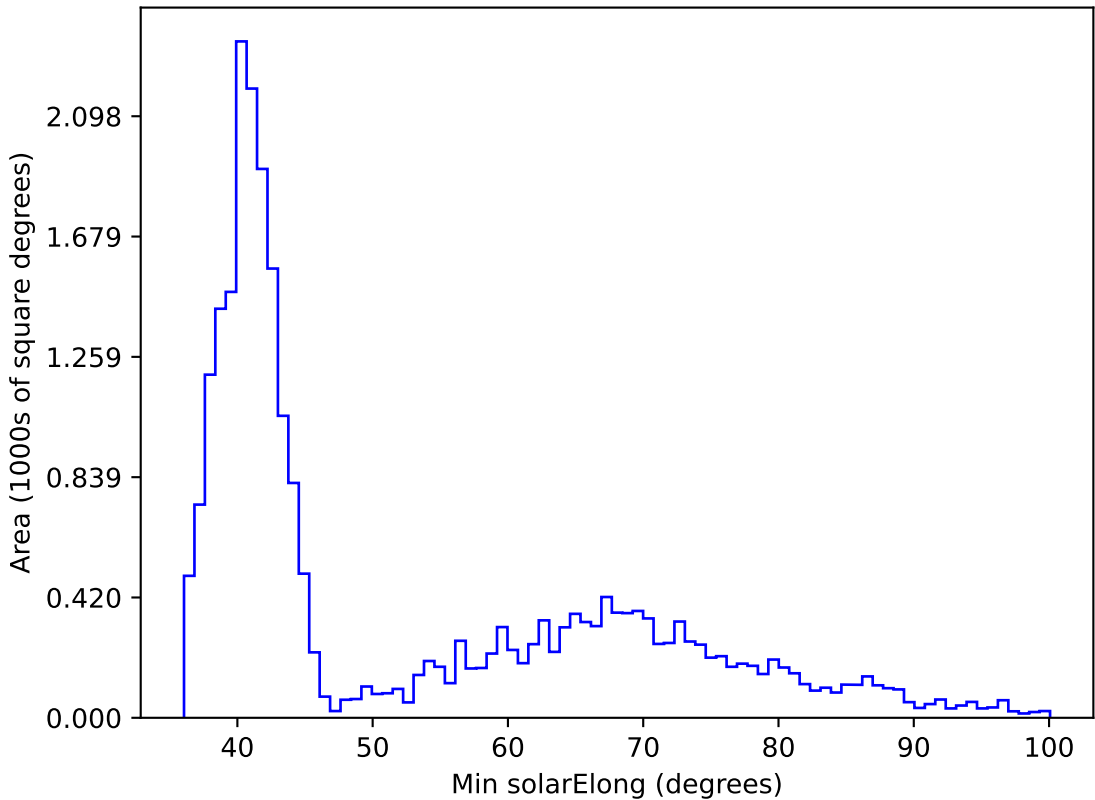
too_elab_r256_d3_ugrizy_v3.4_10yrs All sky i band: Min solarElong
