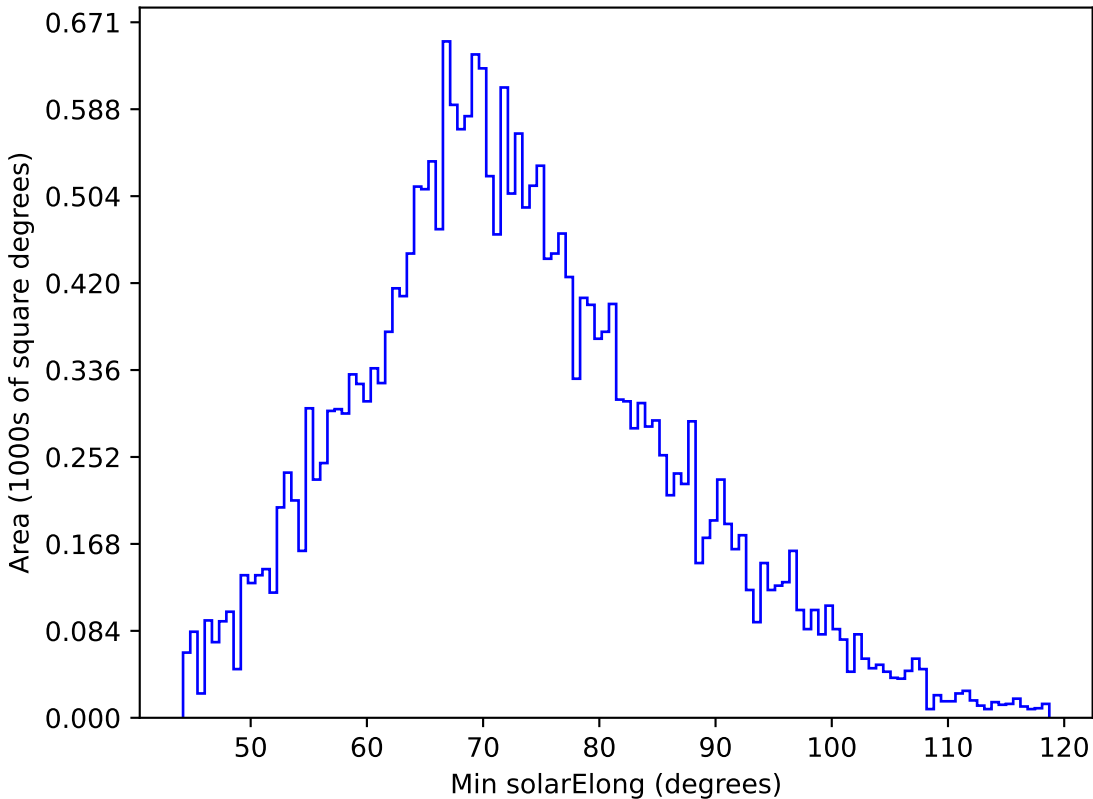
too_elab_r256_d3_ugrizy_v3.4_10yrs All sky g band: Min solarElong
