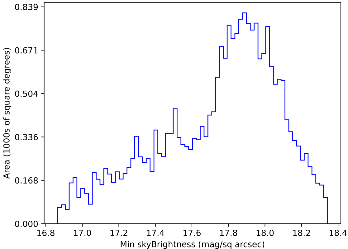
too_elab_r256_d3_ugrizy_v3.4_10yrs Yr 1 y band: Min skyBrightness
