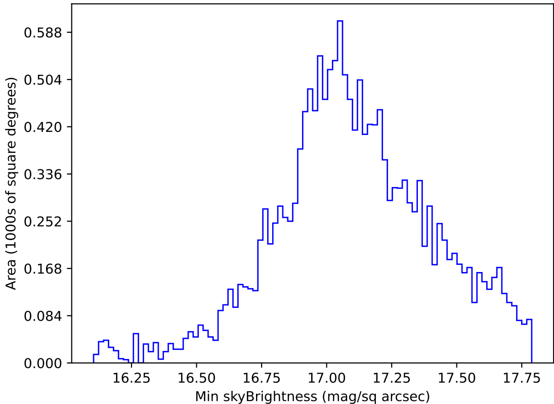
too_elab_r256_d3_ugrizy_v3.4_10yrs WFD y band: Min skyBrightness
