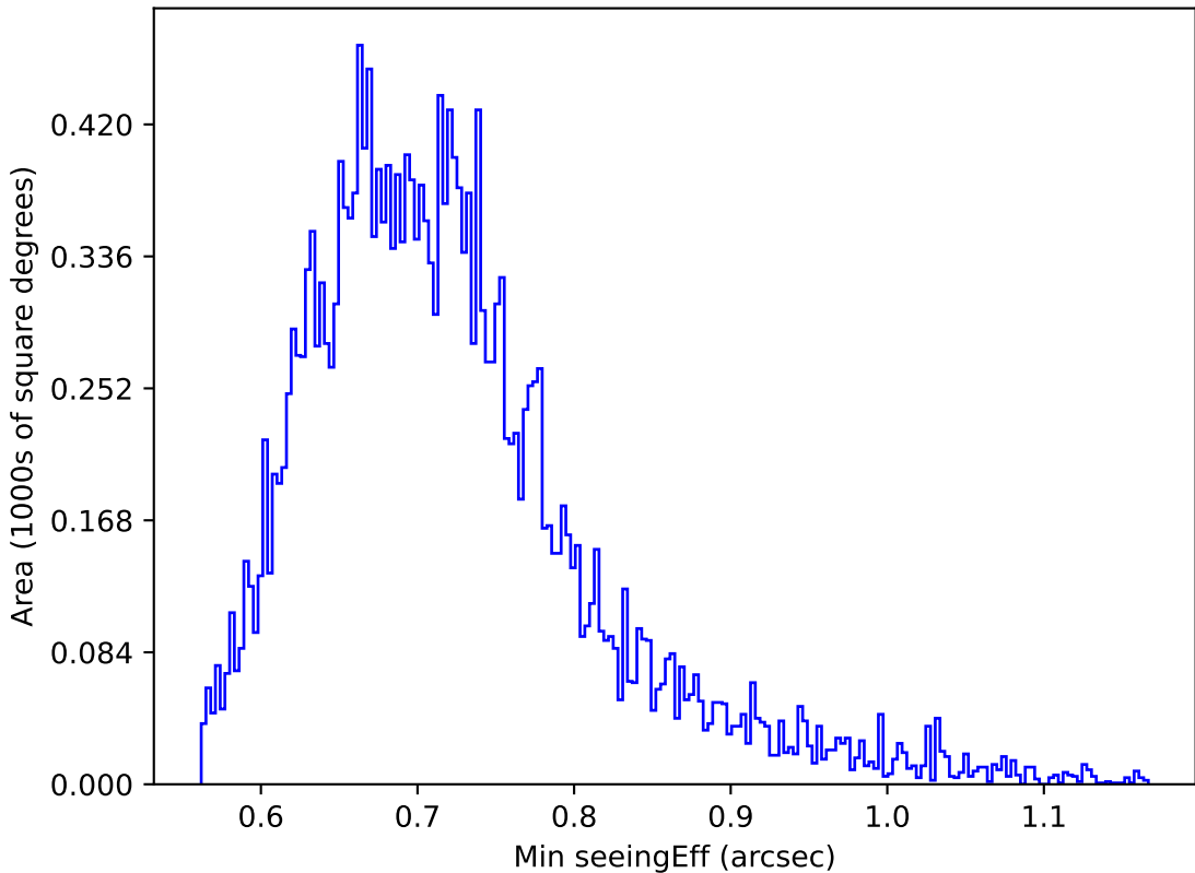
too_elab_r256_d3_ugrizy_v3.4_10yrs Yr 1 y band: Min seeingEff
