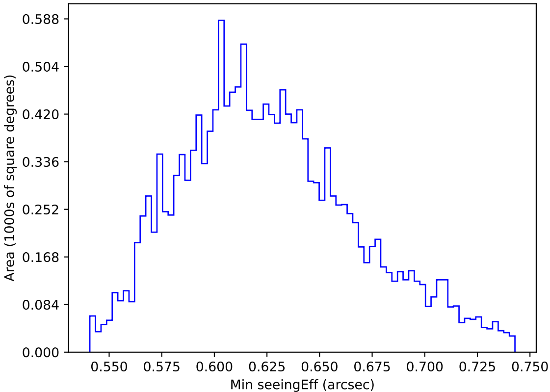
too_elab_r256_d3_ugrizy_v3.4_10yrs WFD y band: Min seeingEff
