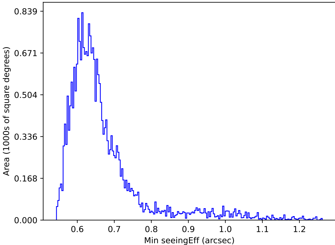
too_elab_r256_d3_ugrizy_v3.4_10yrs All sky y band: Min seeingEff
