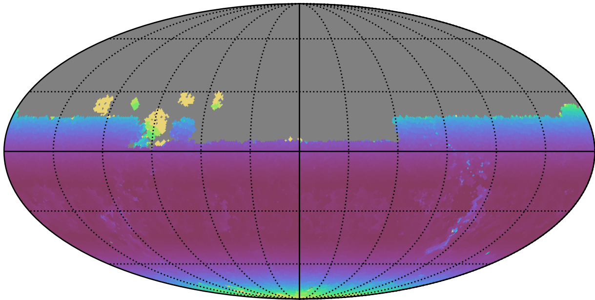
too_elab_r256_d3_ugrizy_v3.4_10yrs Yr 1 y band: Min airmass
