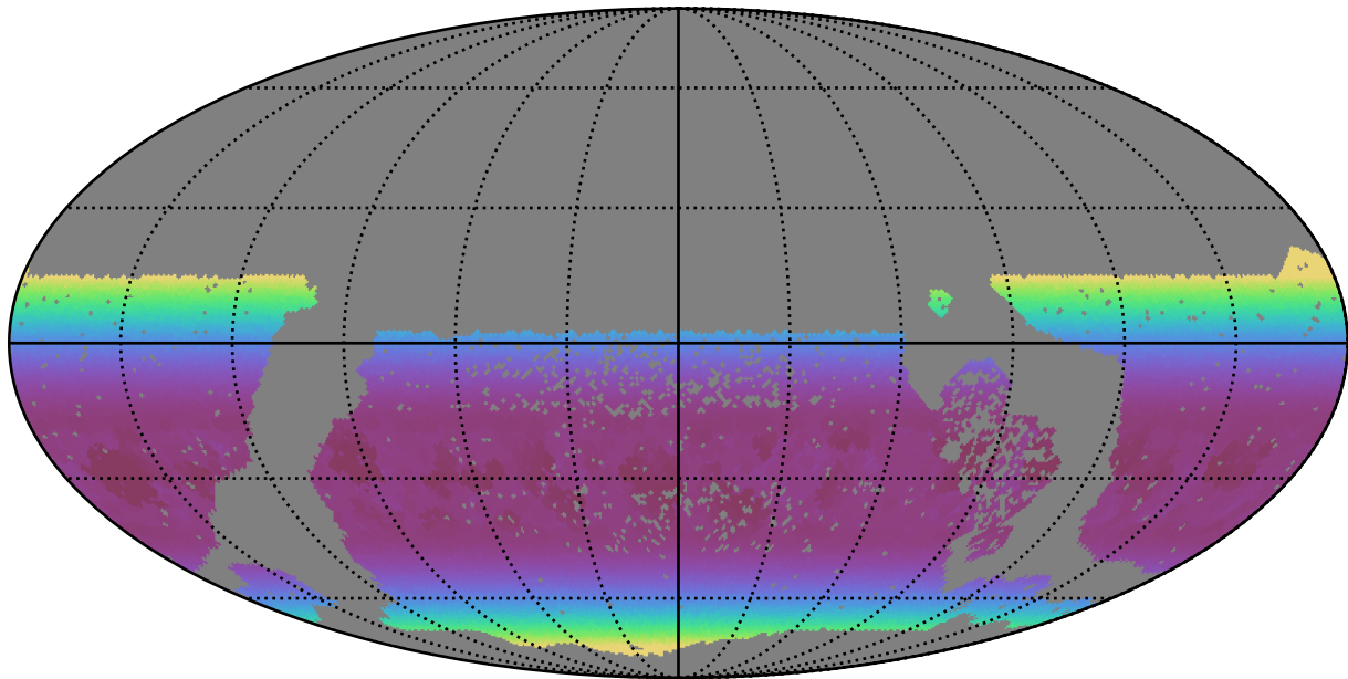
too_elab_r256_d3_ugrizy_v3.4_10yrs WFD y band: Min airmass
