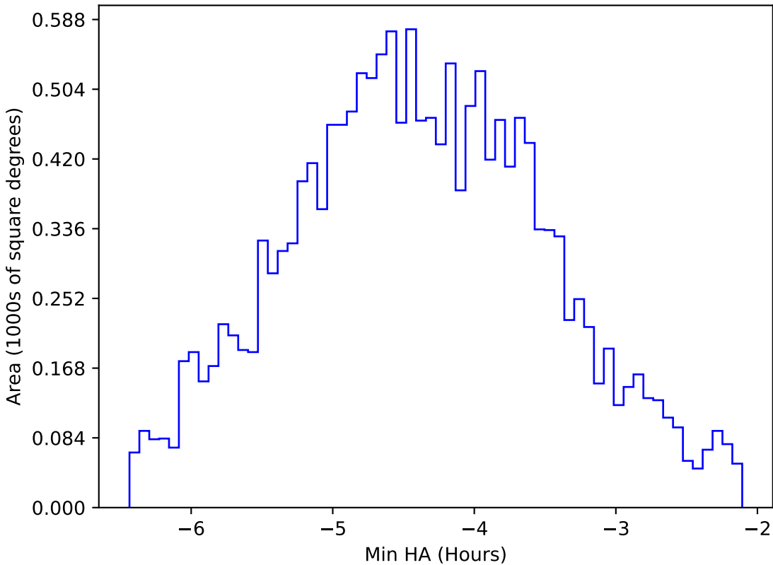
too_elab_r256_d3_ugrizy_v3.4_10yrs WFD z band: Min HA
