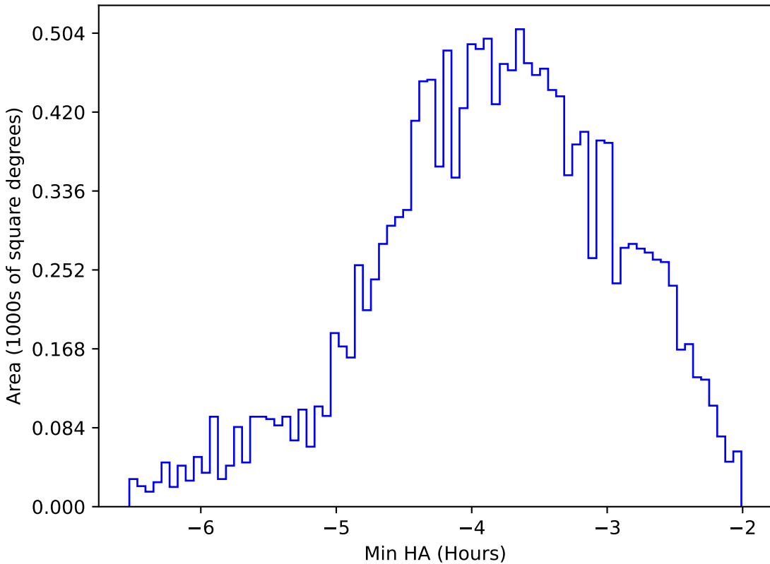
too_elab_r256_d3_ugrizy_v3.4_10yrs WFD y band: Min HA
