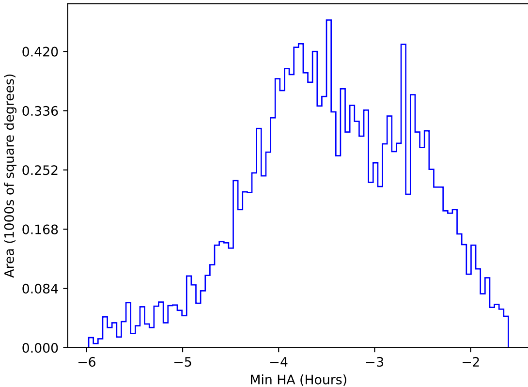
too_elab_r256_d3_ugrizy_v3.4_10yrs WFD u band: Min HA
