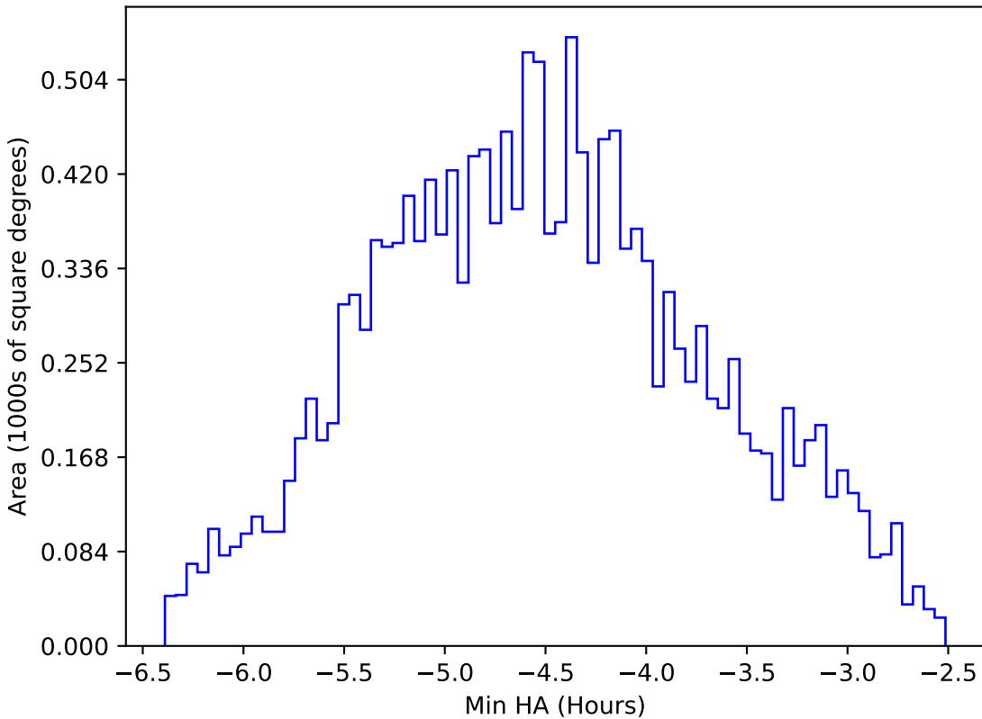
too_elab_r256_d3_ugrizy_v3.4_10yrs WFD r band: Min HA
