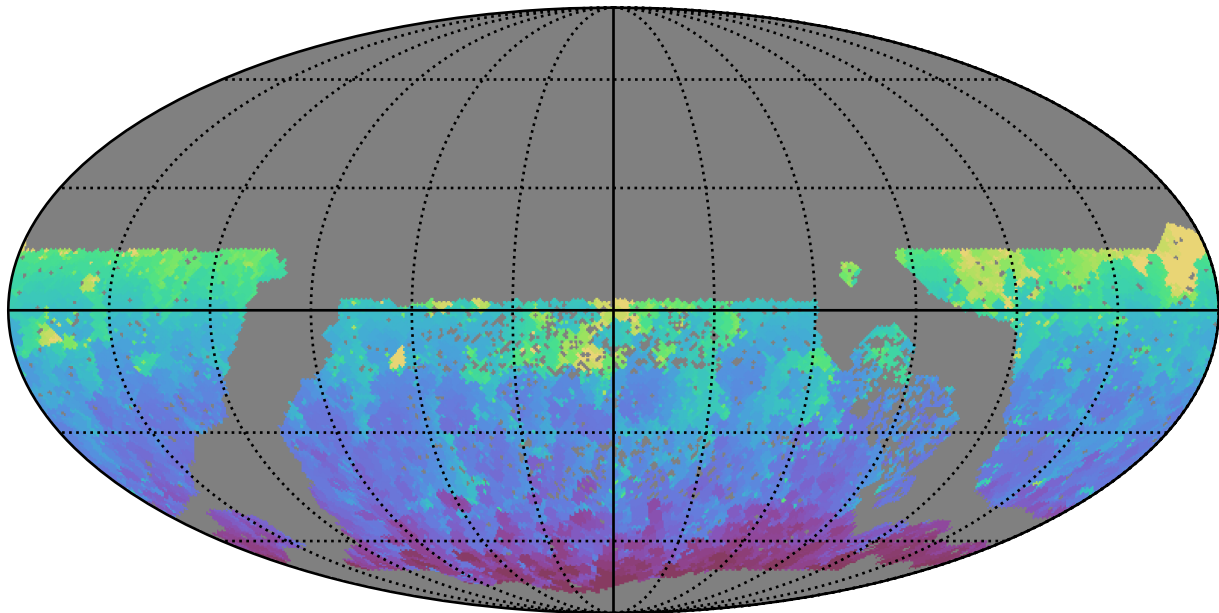
too_elab_r256_d3_ugrizy_v3.4_10yrs WFD g band: Min HA
