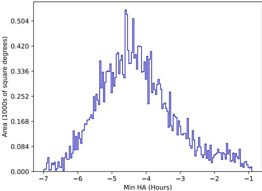
too_elab_r256_d3_ugrizy_v3.4_10yrs All sky r band: Min HA
