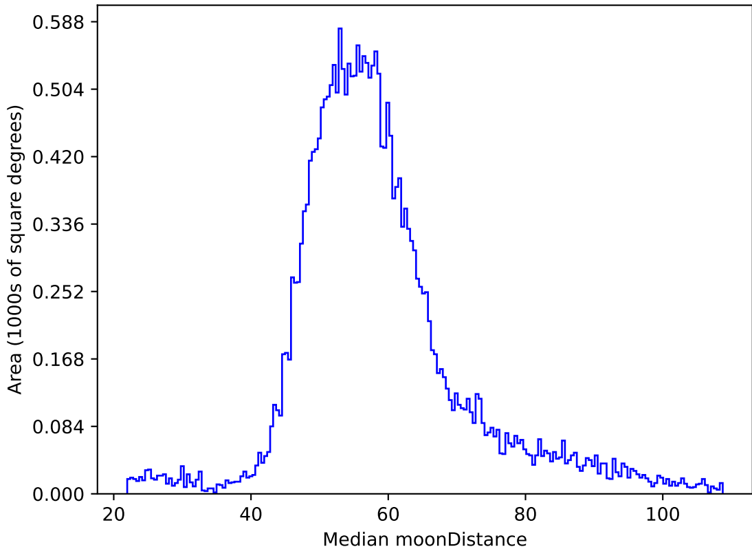
too_elab_r256_d3_ugrizy_v3.4_10yrs All sky y band: Median moonDistance
