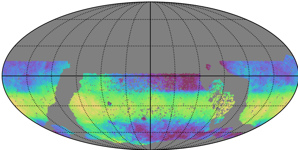
too_elab_r256_d3_ugrizy_v3.4_10yrs WFD y band: Median HA
