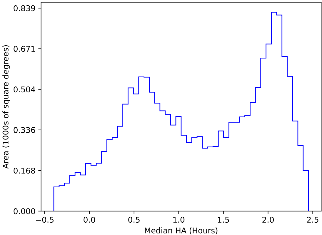
too_elab_r256_d3_ugrizy_v3.4_10yrs WFD y band: Median HA
