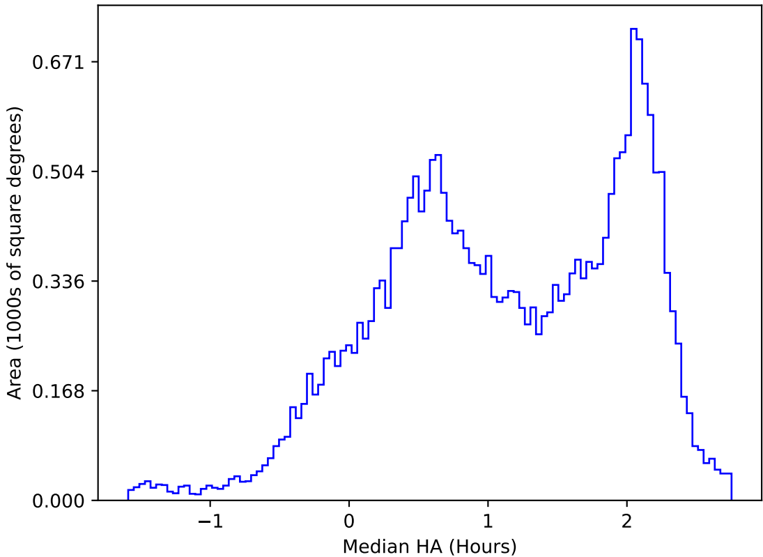
too_elab_r256_d3_ugrizy_v3.4_10yrs All sky y band: Median HA
