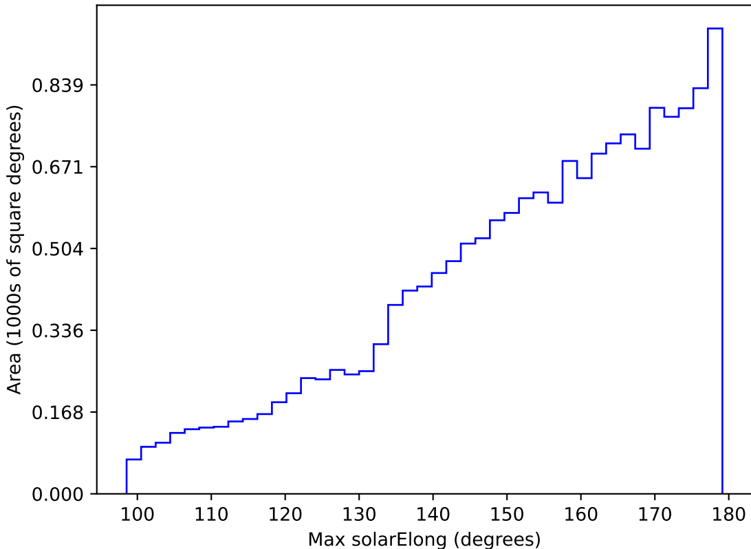
too_elab_r256_d3_ugrizy_v3.4_10yrs WFD y band: Max solarElong
