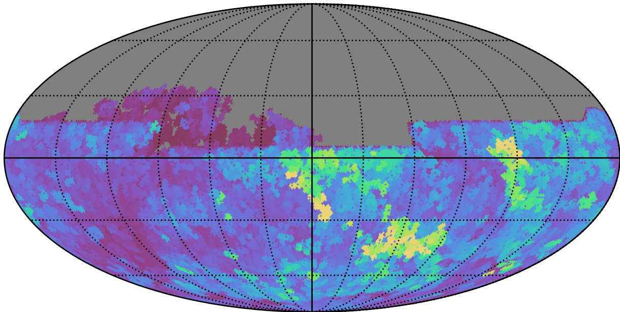
too_elab_r256_d3_ugrizy_v3.4_10yrs All sky y band: Max seeingEff
