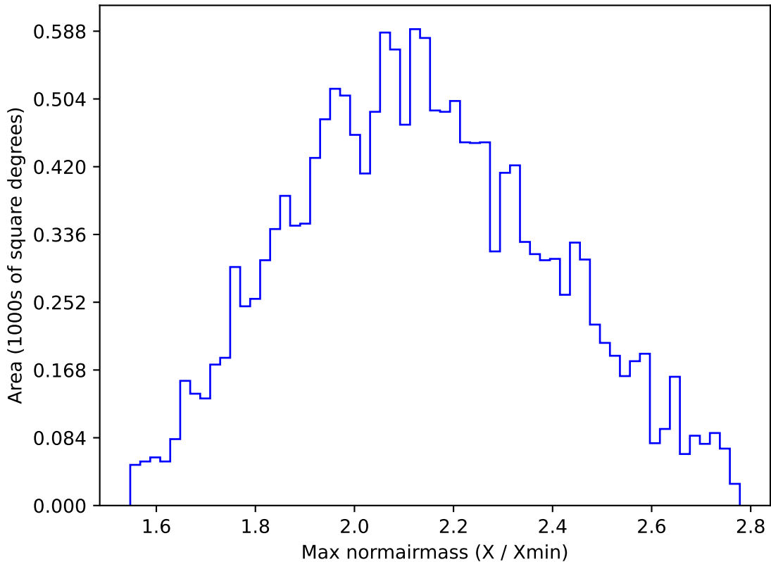
too_elab_r256_d3_ugrizy_v3.4_10yrs WFD y band: Max normairmass
