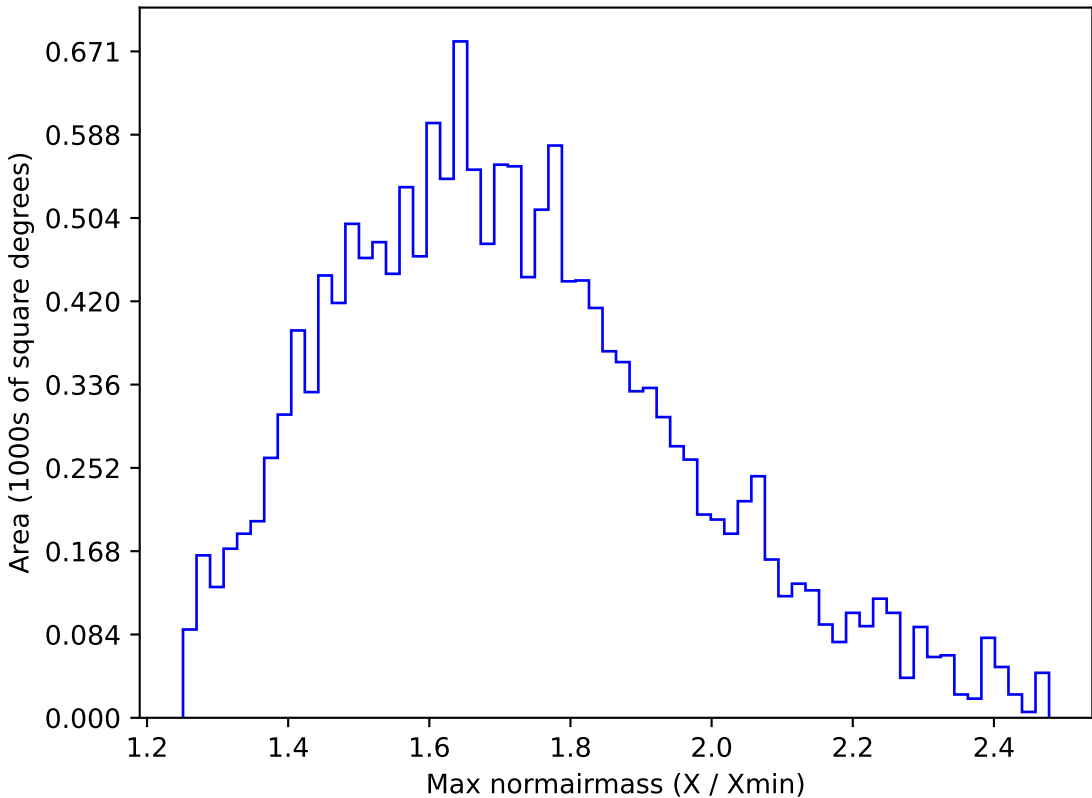
too_elab_r256_d3_ugrizy_v3.4_10yrs WFD u band: Max normairmass
