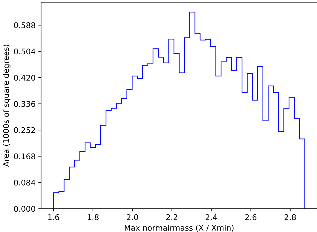
too_elab_r256_d3_ugrizy_v3.4_10yrs WFD i band: Max normairmass
