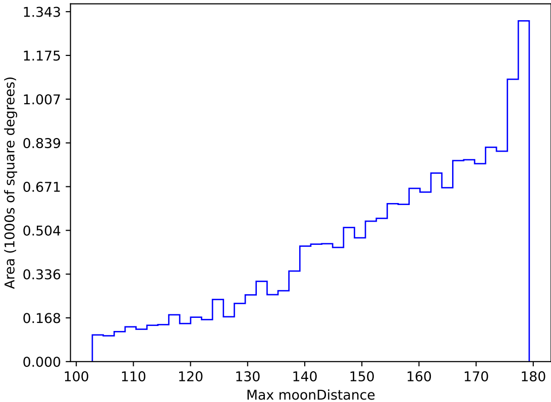
too_elab_r256_d3_ugrizy_v3.4_10yrs WFD i band: Max moonDistance
