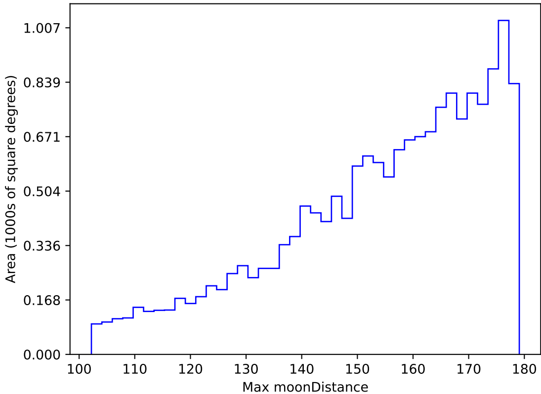
too_elab_r256_d3_ugrizy_v3.4_10yrs WFD g band: Max moonDistance
