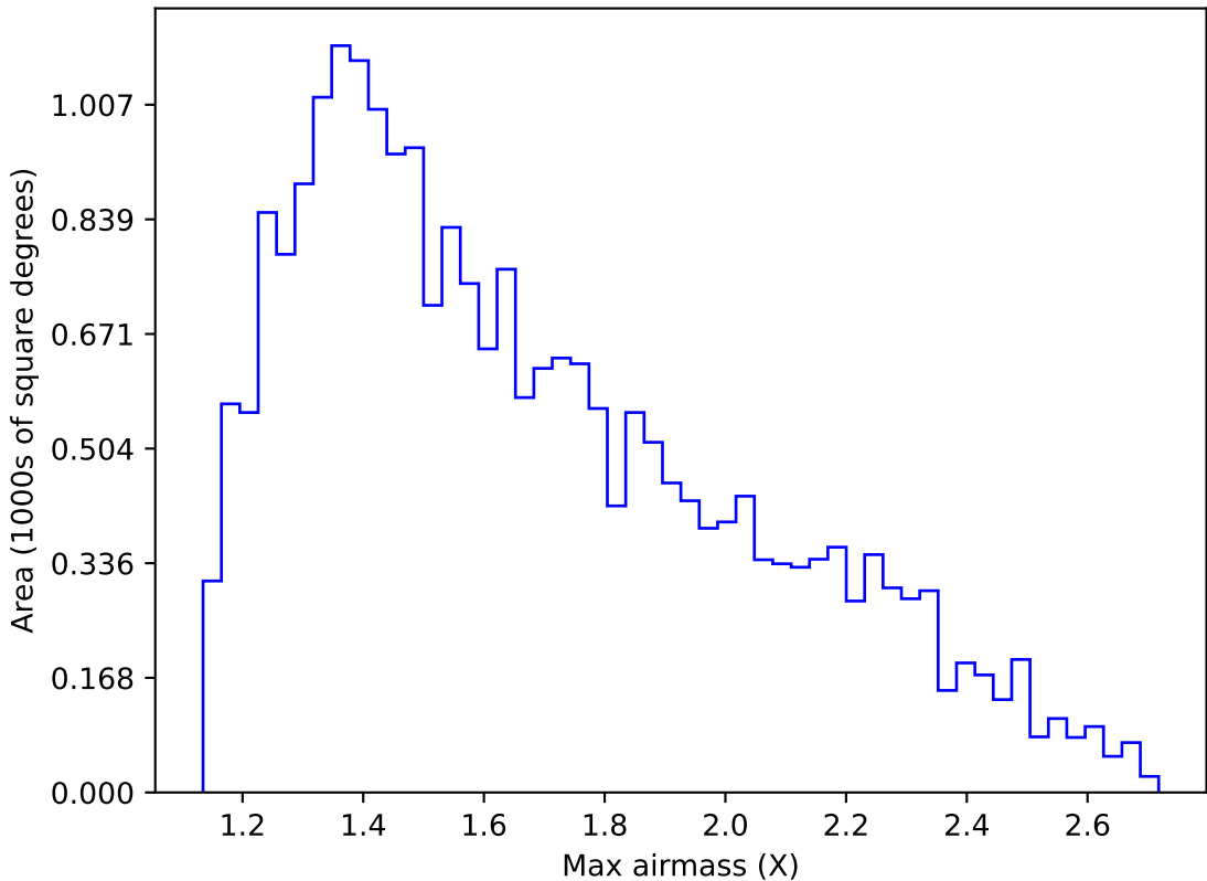
too_elab_r256_d3_ugrizy_v3.4_10yrs Yr 1 y band: Max airmass
