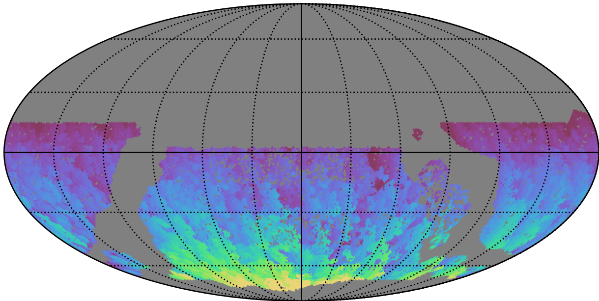
too_elab_r256_d3_ugrizy_v3.4_10yrs WFD y band: Max HA
