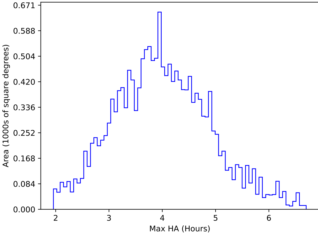
too_elab_r256_d3_ugrizy_v3.4_10yrs WFD u band: Max HA
