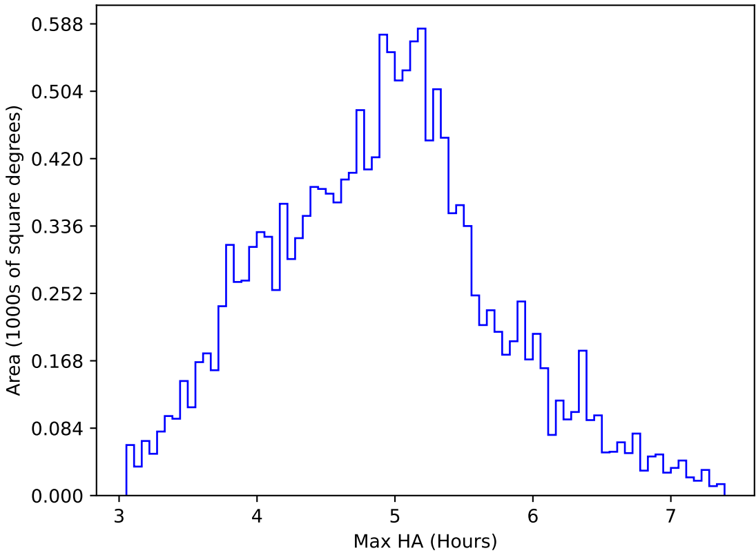
too_elab_r256_d3_ugrizy_v3.4_10yrs WFD i band: Max HA
