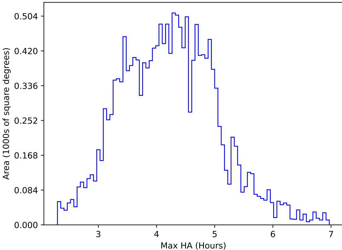
too_elab_r256_d3_ugrizy_v3.4_10yrs WFD g band: Max HA
