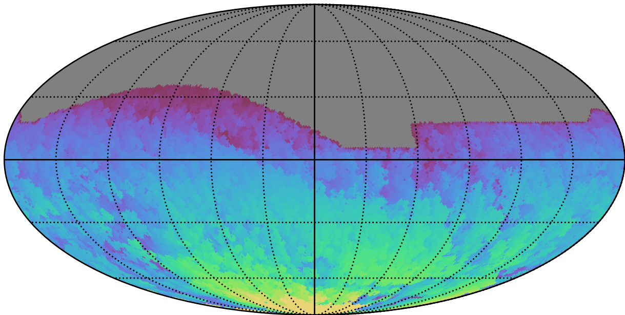
too_elab_r256_d3_ugrizy_v3.4_10yrs All sky z band: Max HA
