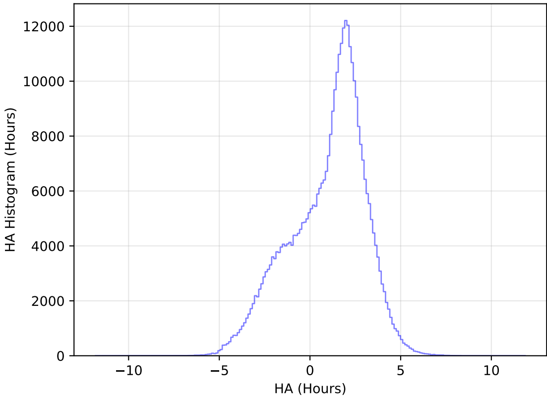
too_elab_r256_d3_ugrizy_v3.4_10yrs All sky y band: HA Histogram
