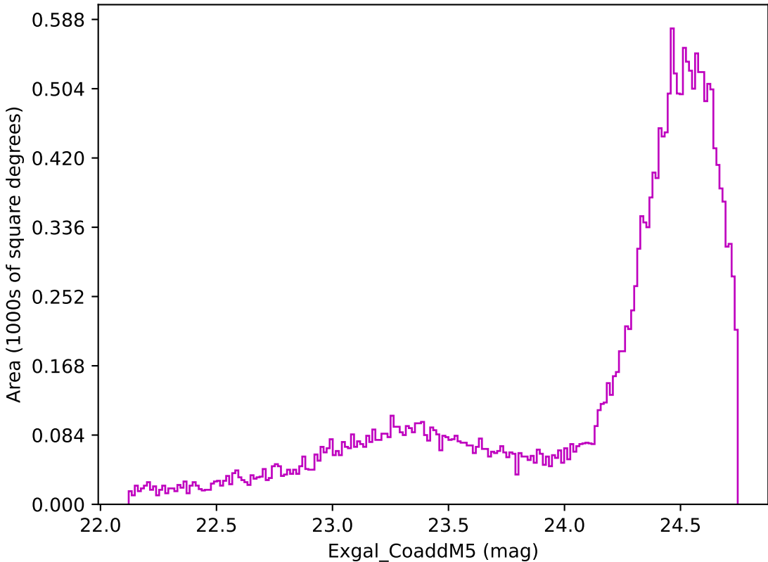
too_elab_r256_d3_ugrizy_v3.4_10yrs Yr 1 z band: Exgal_CoaddM5
